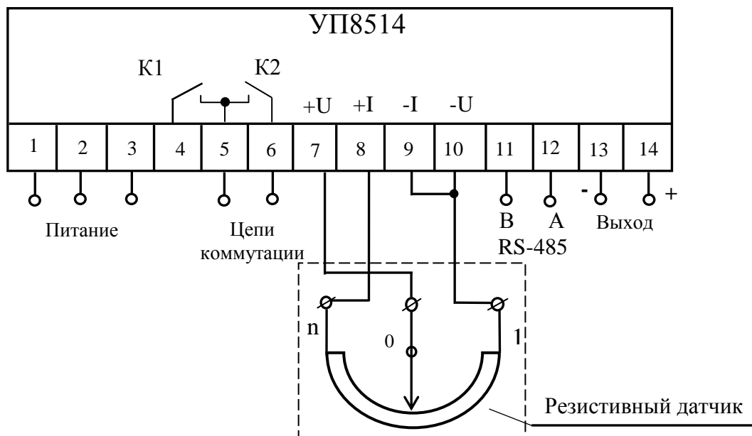
Рисунок Д.3 – Схема электрическая подключения указателей УП8514/1, УП8514/2 с габаритными размерами 96x96x130 mm при трехпроводном подключении резистивного датчика
