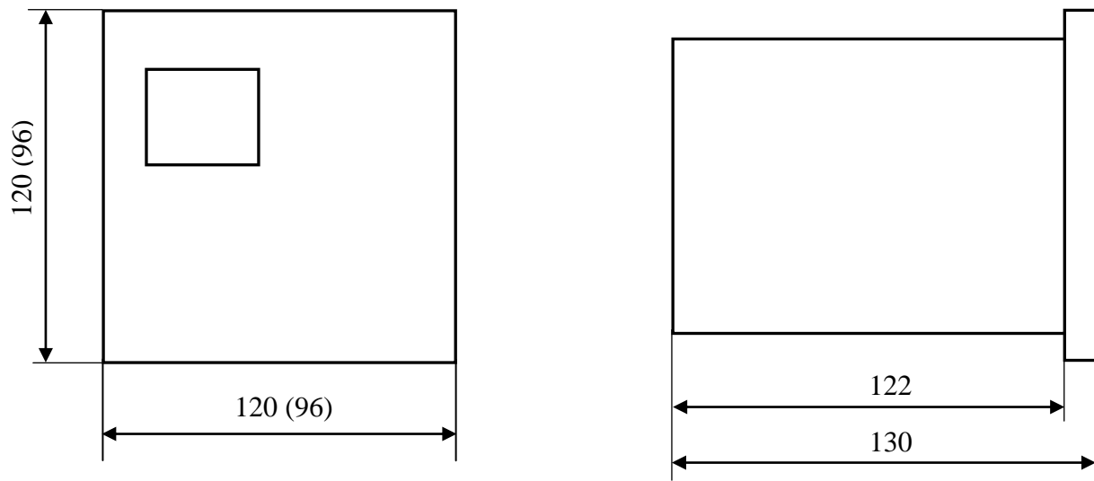
Рисунок Г.1 – Габаритные размеры указателя
