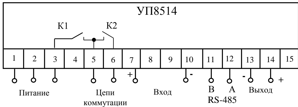
Рисунок Е.1 – Схема электрическая подключения указателей УП8514/3-УП8514/6 с габаритными размерами 120x120x130 mm
