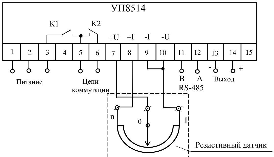
Рисунок Д.1 – Схема электрическая подключения указателей УП8514/1, УП8514/2 с габаритными размерами 120x120x130 mm при трехпроводном подключении резистивного датчика
