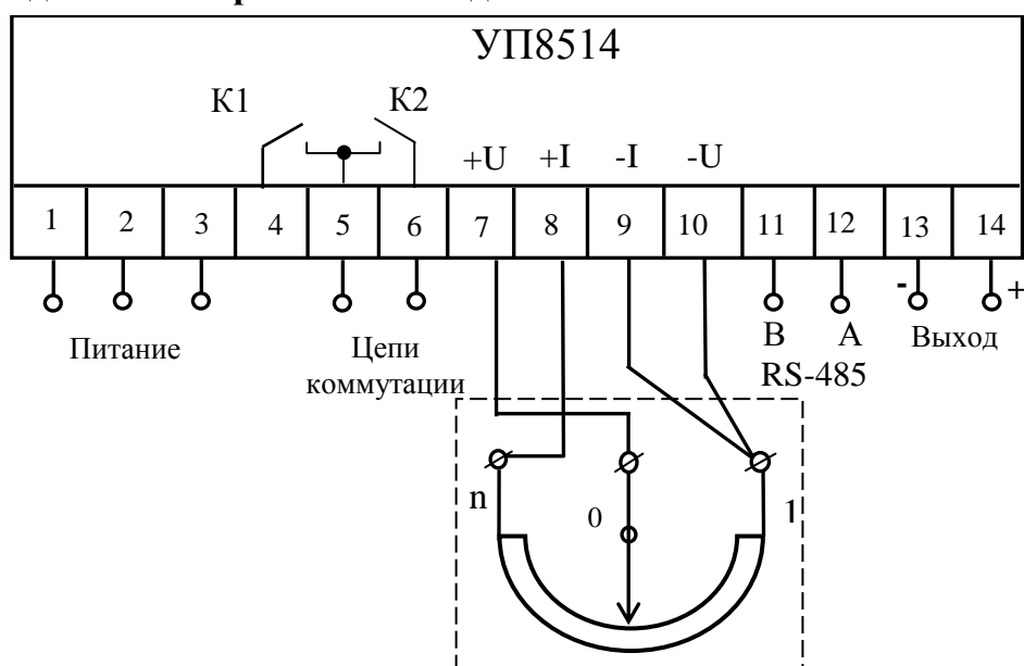
Рисунок Д.4 – Схема электрическая подключения указателей УП8514/1, УП8514/2 с габаритными размерами 96x96x130 mm при четырехпроводном подключении резистивного датчика
