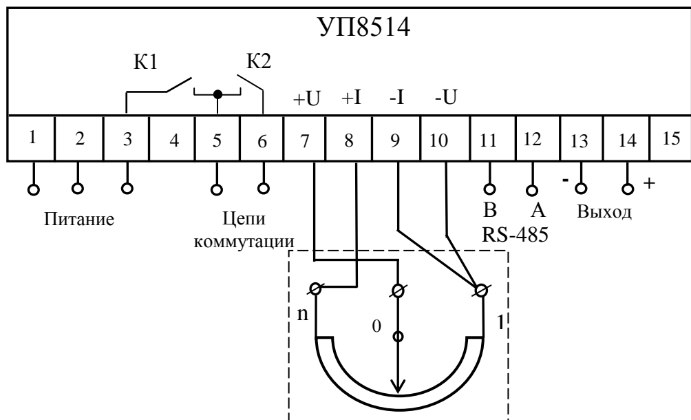
Рисунок Д.2 – Схема электрическая подключения указателей УП8514/1, УП8514/2 с габаритными размерами 120x120x130 mm при четырехпроводном подключении резистивного датчика
