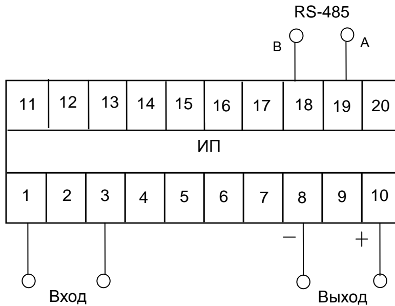
Рисунок Г.1 – Схема подключения ИП ЭП8528/1– ЭП8528/7
