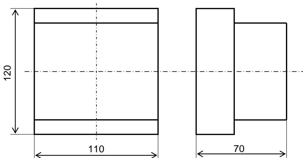
Рисунок В.1– Габаритные размеры ИП
