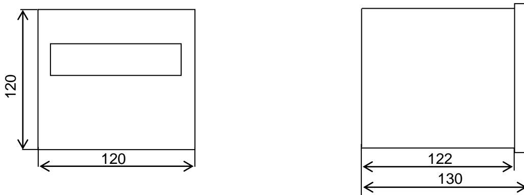
Рисунок Б.1 – Габаритные размеры устройств 120x120x130 мм
