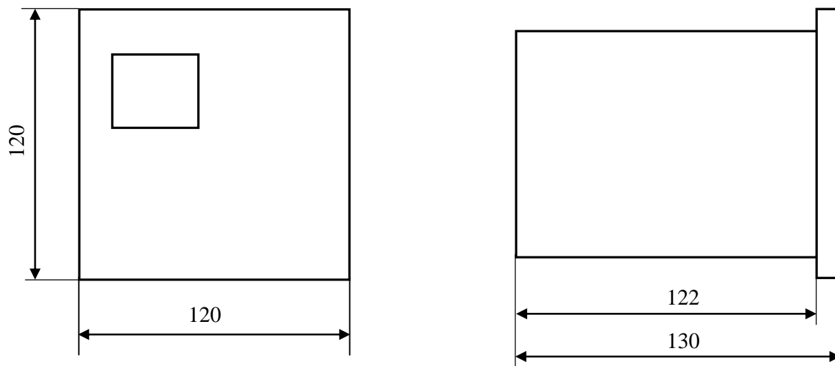
Рисунок В.1 – Габаритные размеры указателя
