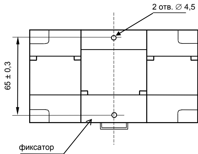
Рисунок В.8 – Установочные размеры ЦП8507/3 – ЦП8507/6
