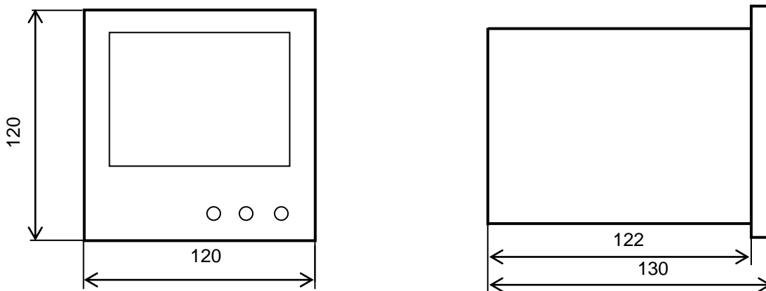
Рисунок В.1 - Габаритные размеры ЦП8507/1, ЦП8507/2
