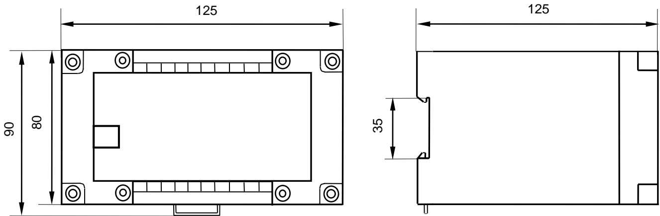
Рисунок В.7 – Габаритные размеры ЦП8507/3 – ЦП8507/6
